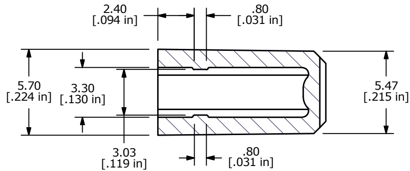
SECTION A-A SCALE 4 : 1
